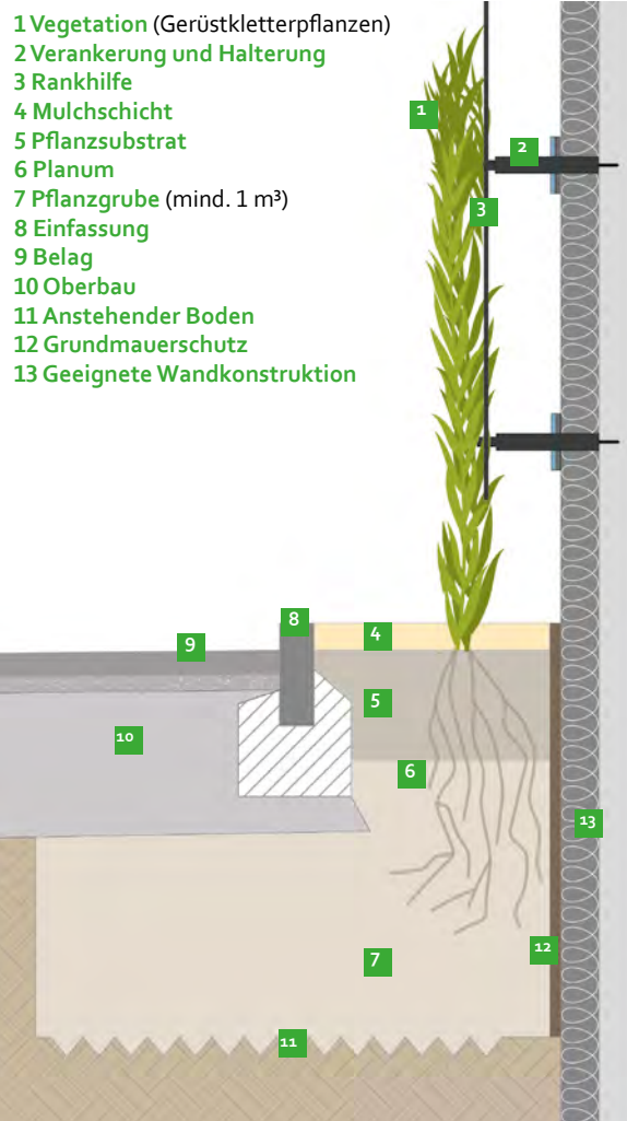
Abb. 45: Grafischer Schnitt einer bodengebundenen Fassadenbegrünung. Quelle: BuGG
