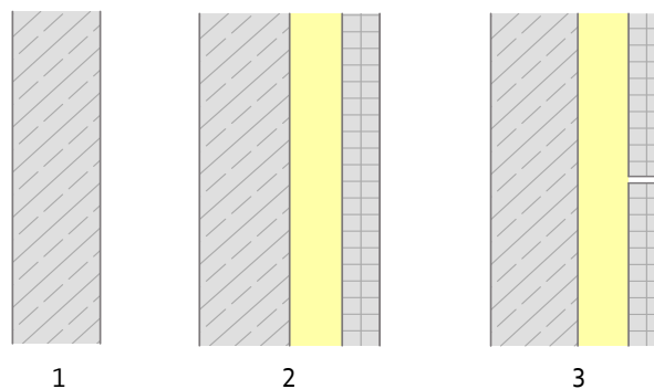
Abb. 170: Sichtbetonbauweisen als exemplarische Vertikalschnitte (Auswahl). Quelle: BuGG
