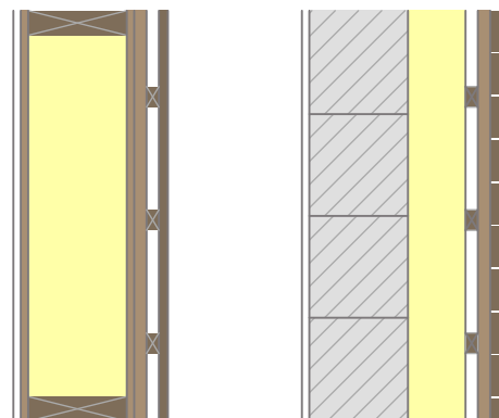
Abb. 188: Vorgehängt hinterlüftete Fassaden als exemplarische Vertikalschnitte (Auswahl). Quelle: BuGG
