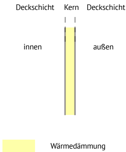
Abb. 182: Vertikalschnitt Sandwichelement. Quelle: BuGG
